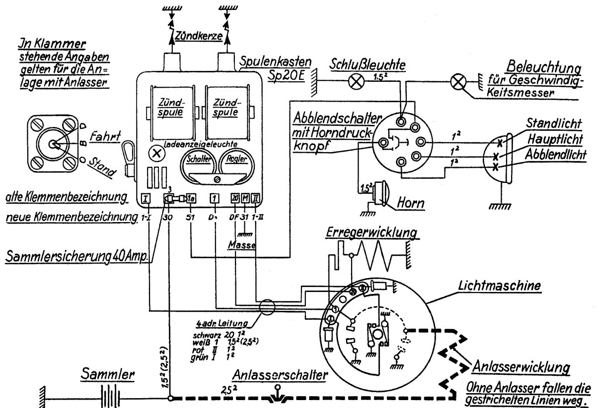
Schaltbild SB 500 mit Spulenkasten Sp 20 E
