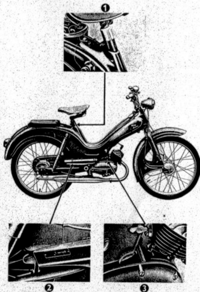
Motor- ② und Fahrgestell-Nummer ③ sowie Typenschild ① der DKW Hummel
