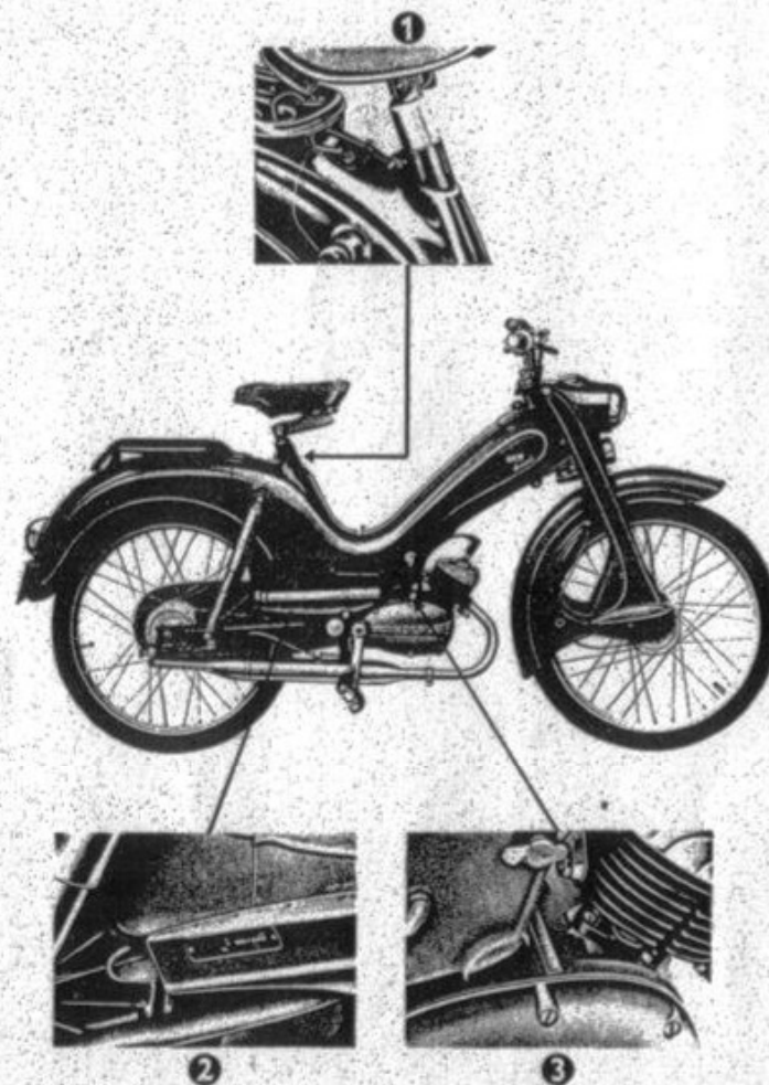
Motor- ② und Fahrgestell-Nummer ③ sowie Typenschild ① der DKW Hummel
