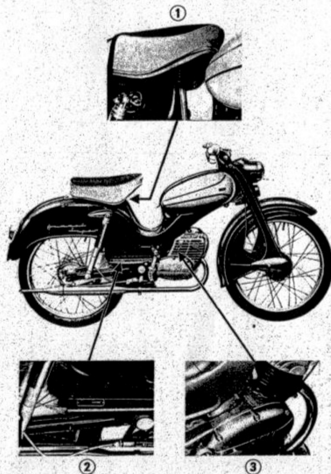
Motor- ① und Fahrgestell-Nummer ② sowie Typenschild ③ der DKW Hummel Super
