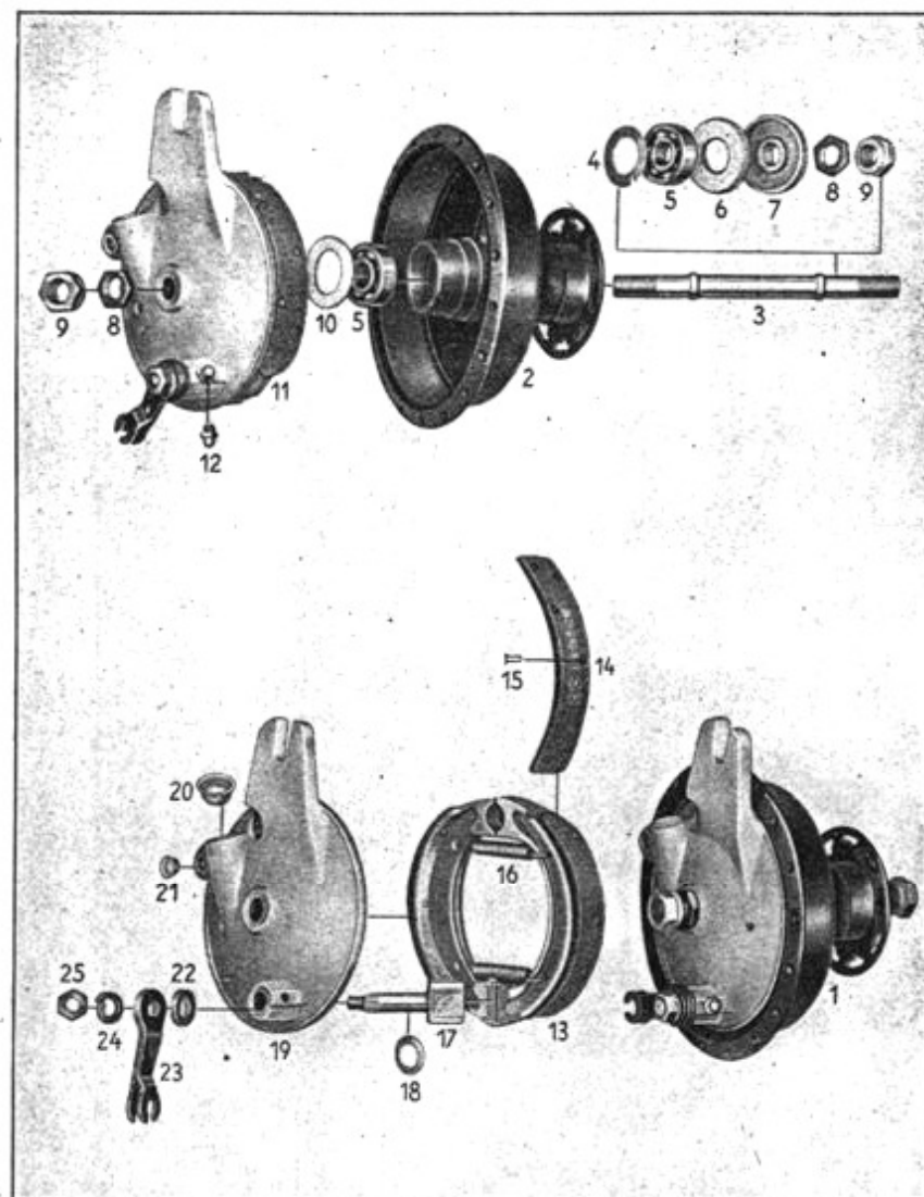
Tafel 22 Gruppe B: b) Vorderradnabe
