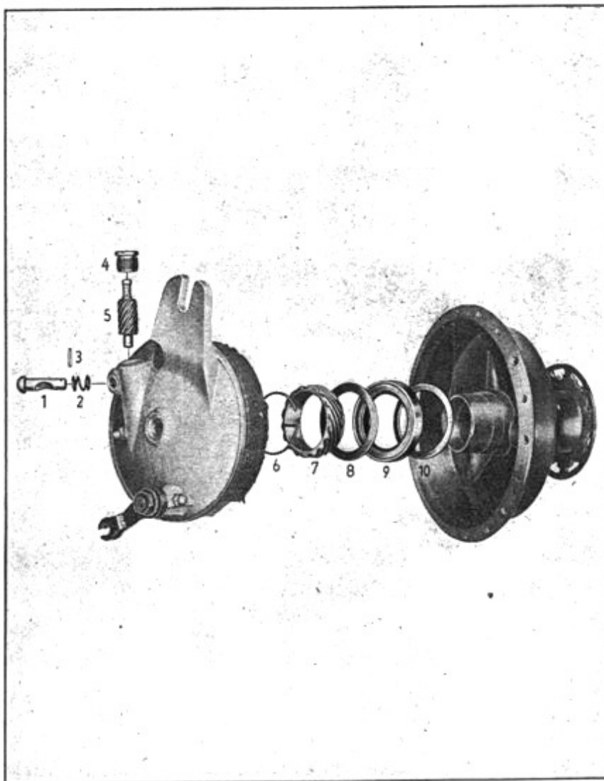
Tafel 33 Gruppe E: b) Antriebsteile für Geschwindigkeitsmesser
