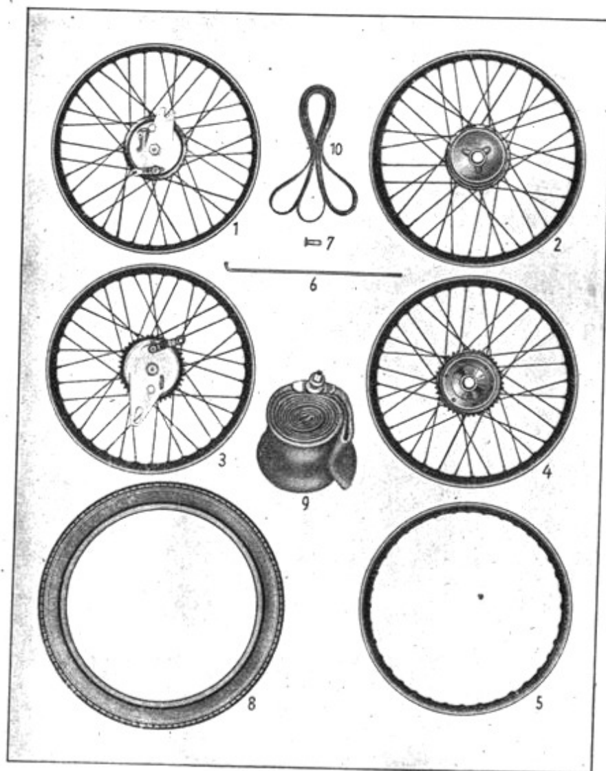
Tafel 21 Gruppe B: b—c) Räder
