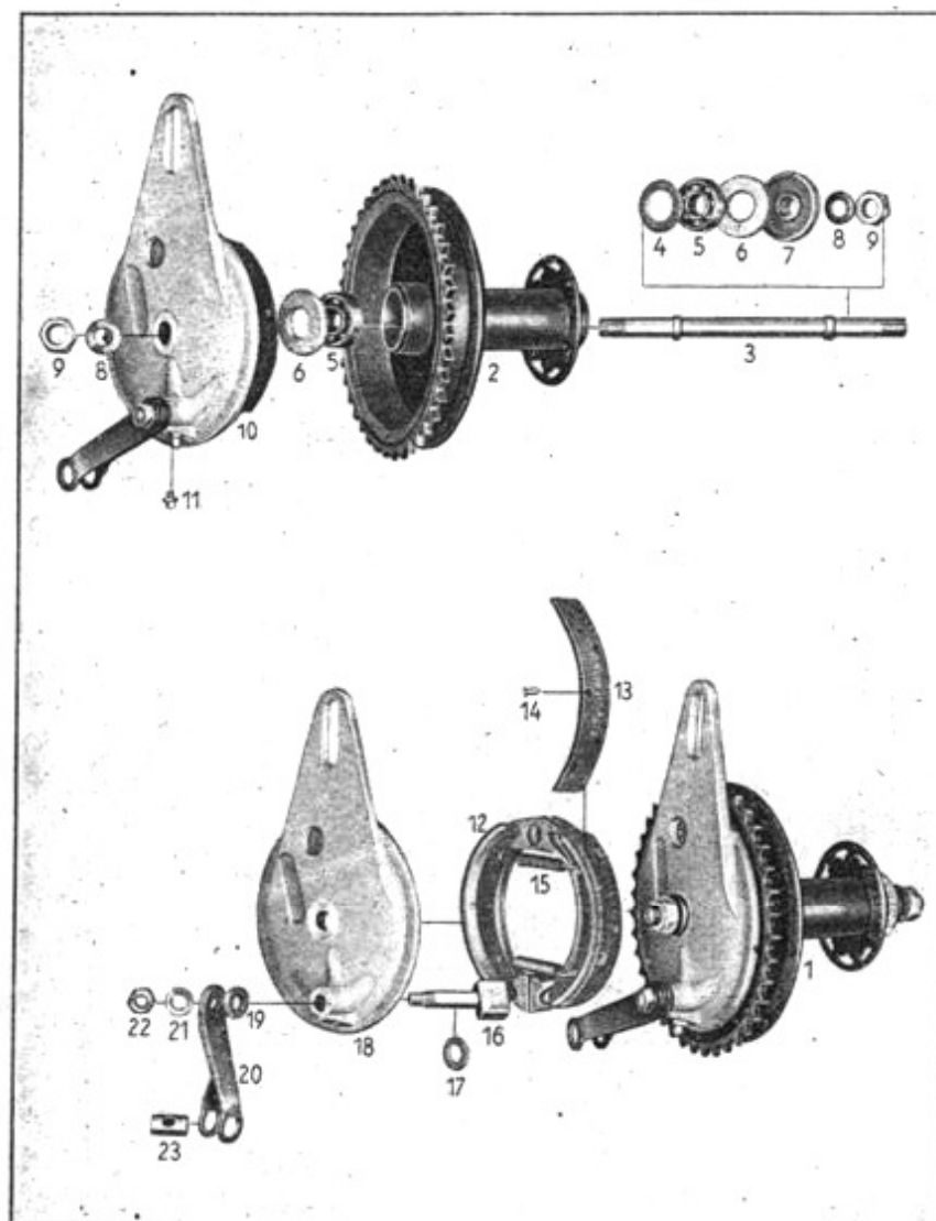
Tafel 23 Gruppe B: c) Hinterradnabe
