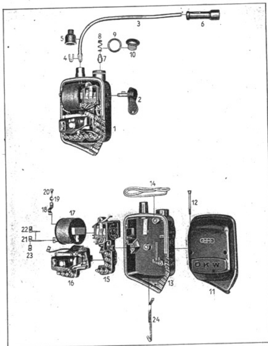
Tafel 28 Gruppe E: Elektrische Ausrüstung, Schaltkasten
