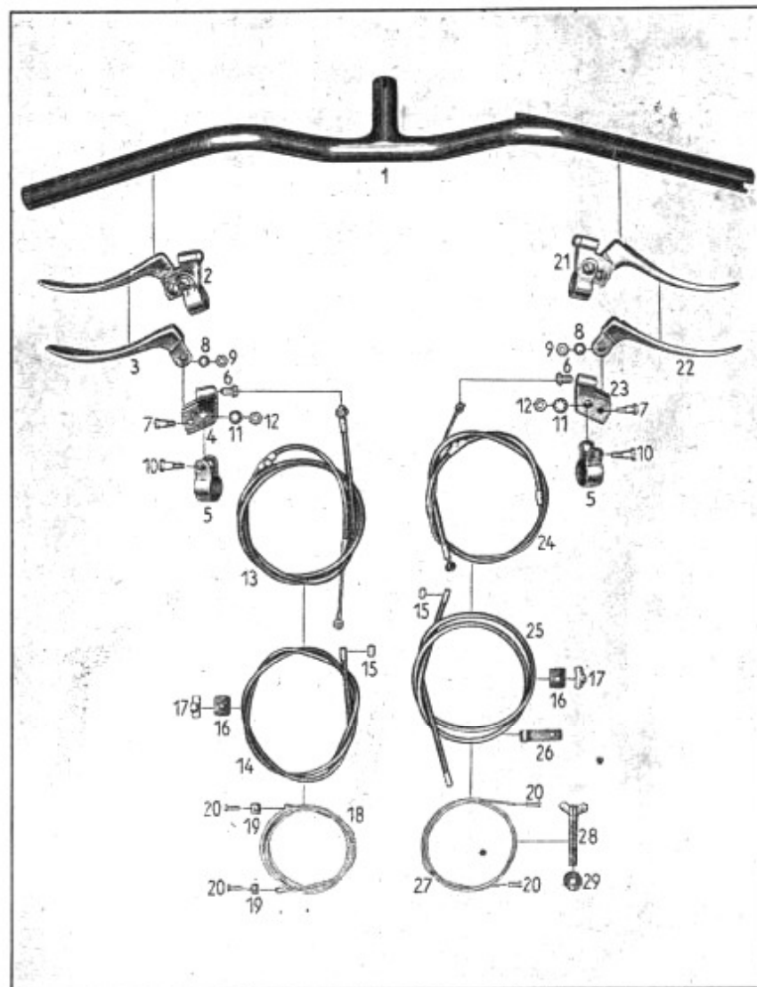
Tafel 19 Gruppe R: k) Lenker mit Betätigungen
