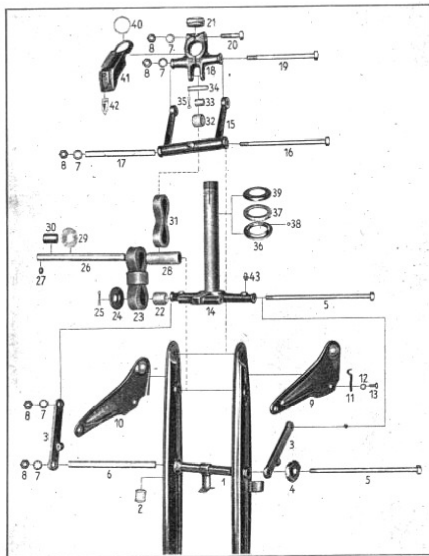
Tafel 18 Gruppe R: i) Federgabel
