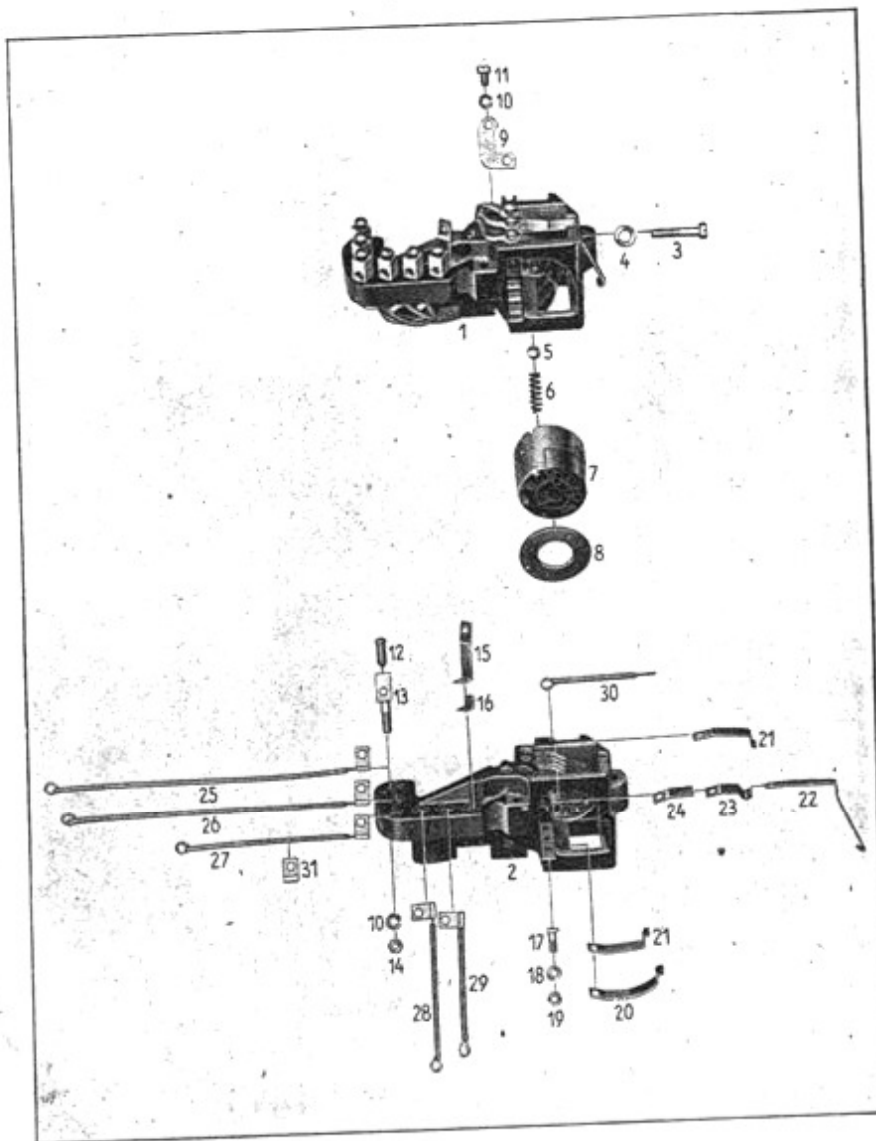
Tafel 29 Gruppe E: Elektrische Ausrüstung: Schaltkasten Klemms- sockel mit Schaltwalzengehäuse
