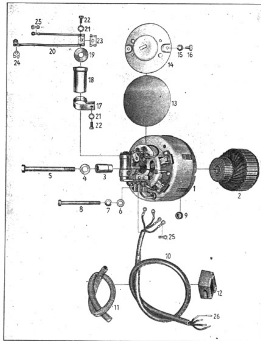
Tafel 25 Gruppe E: Elektrische Ausrüstung, Lichtmaschine, Anker
