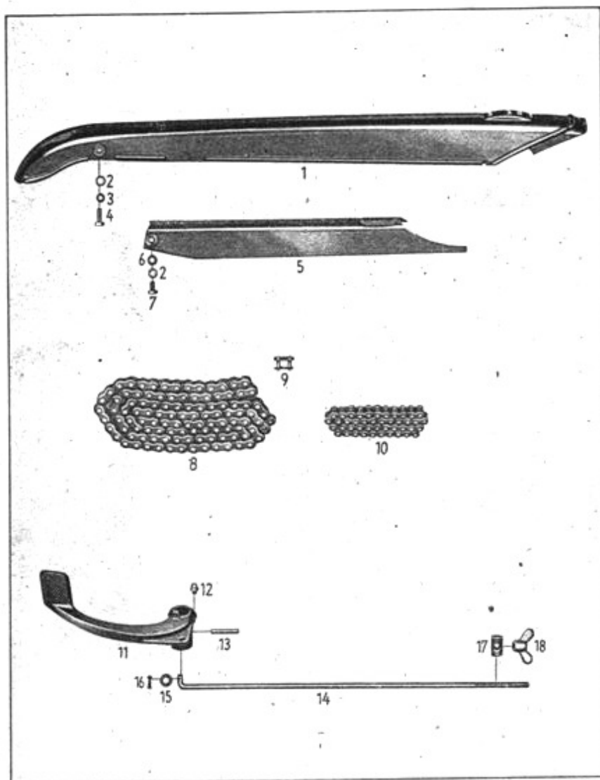
Tafel 24 Gruppe B: a) Fußbremse, d) Antrieb- und Abdeckteile
