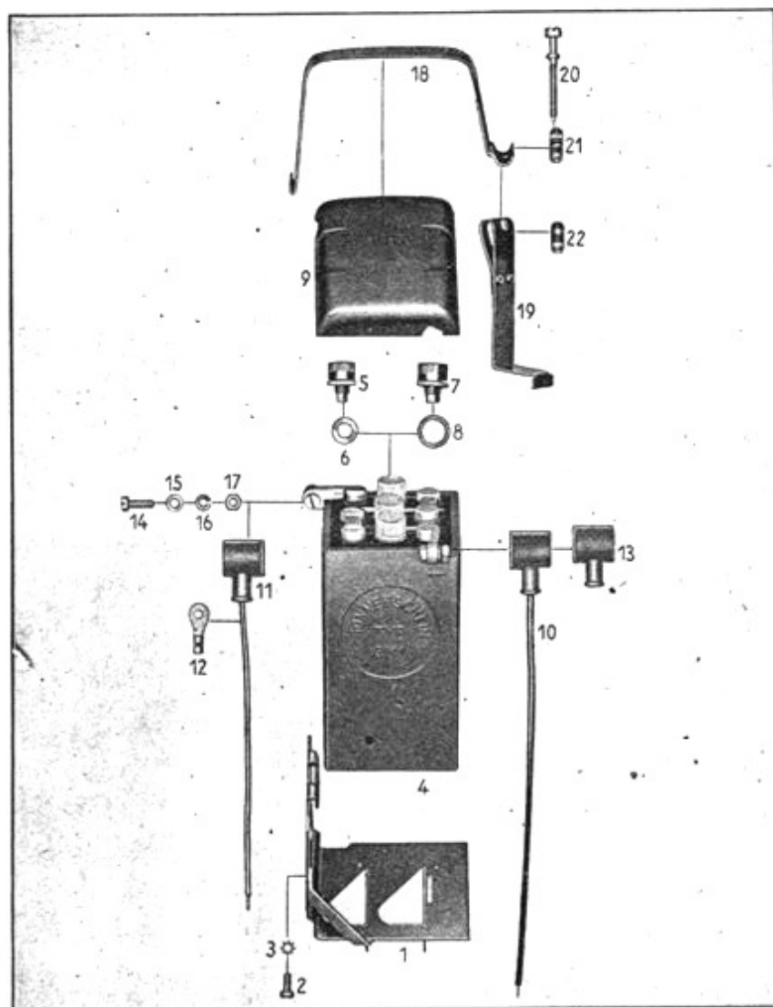
Tafel 27 Gruppe E: Elektrische Ausrüstung, Sammler
