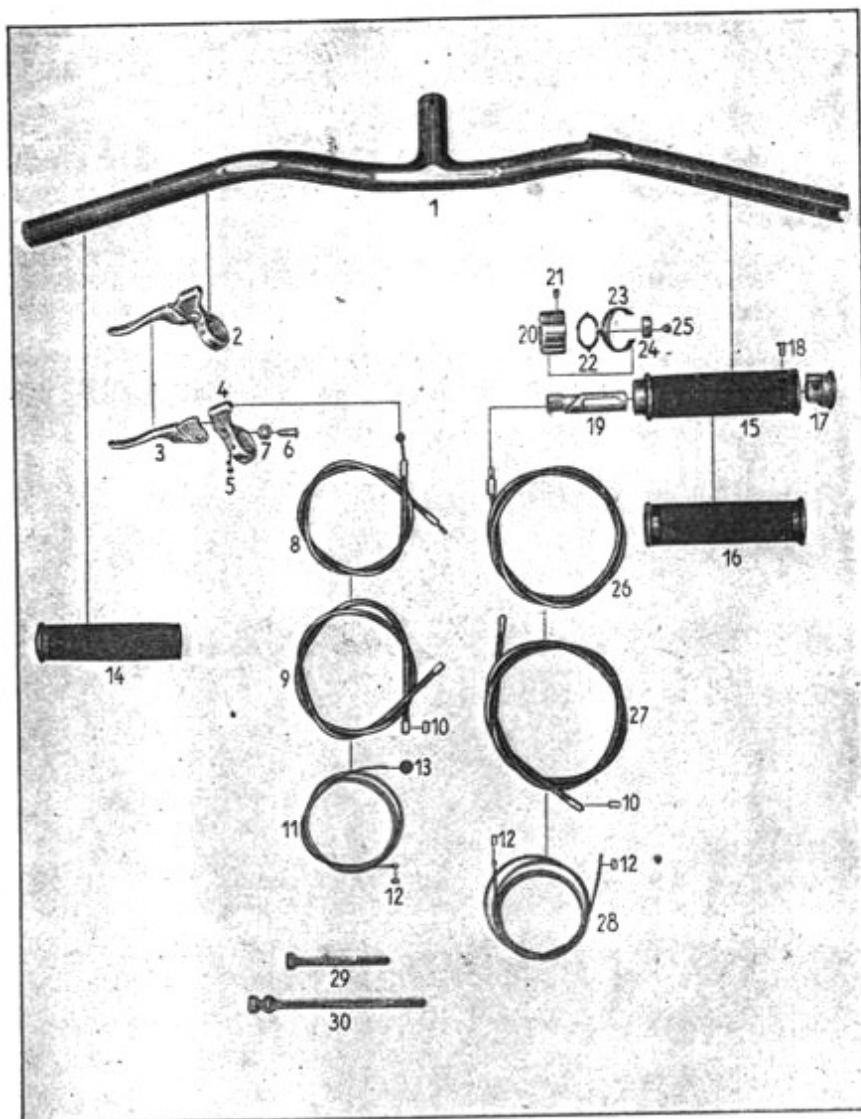
Tafel 20 Gruppe R: k) Lenker mit Betätigungen
