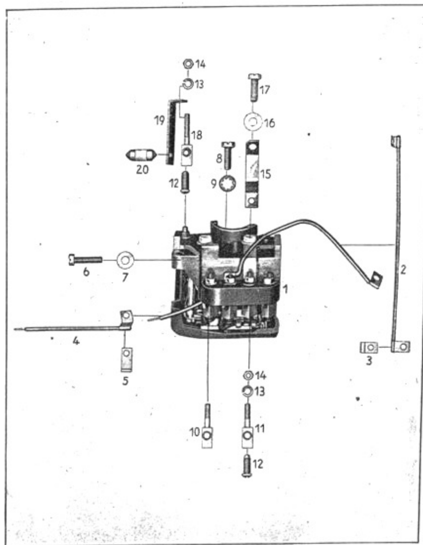
Tafel 30 Gruppe E: Elektrische Ausrüstung, Schaltkasten: Klemmsockel mit Flachreglerschalter
